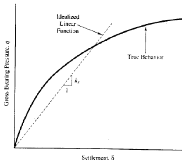
شکل ۲۰- مدل رفتاری تنش-تغییر شکل (واقعی غیرخطی و معادل شده خطی)
