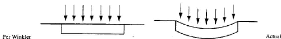
شکل ۲۱- تغییر شکل واقعی پی گسترده غیر صلب و مدل وینکلر
